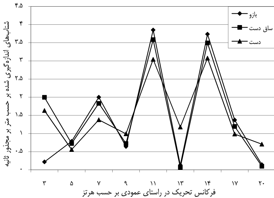
نمودار (۸). میانگین‌های شتاب اندازه‌گیری شده روی دست، بازو و ساق دست در راستای عمودی
