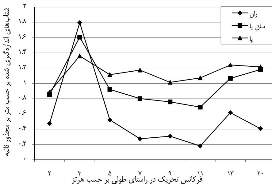
نمودار (۳). میانگین‌های شتاب اندازه‌گیری شده روی ران، پا و ساق آن در راستای طولی
