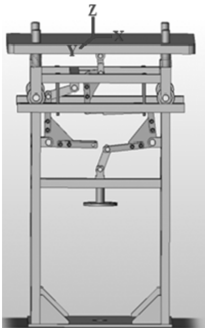
شکل (۱). فیکسچر صندلی تراکتور برای شبیه سازی ارتعاش راننده در راستای طولی، عرضی و عمودی
