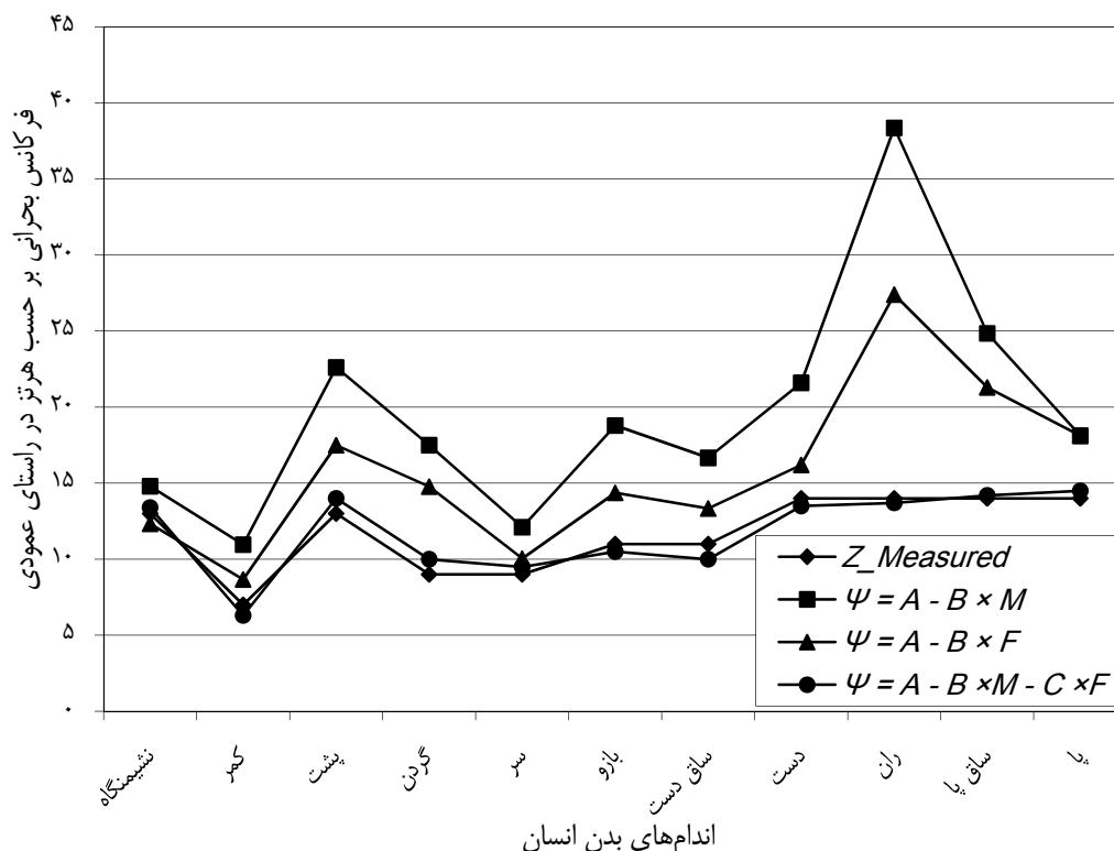
نمودار (۱۲). مقایسه مقادیر فرکانس بحرانی محاسبه و برآوردشده برای اندام‌های بدن انسان در راستای عمودی
