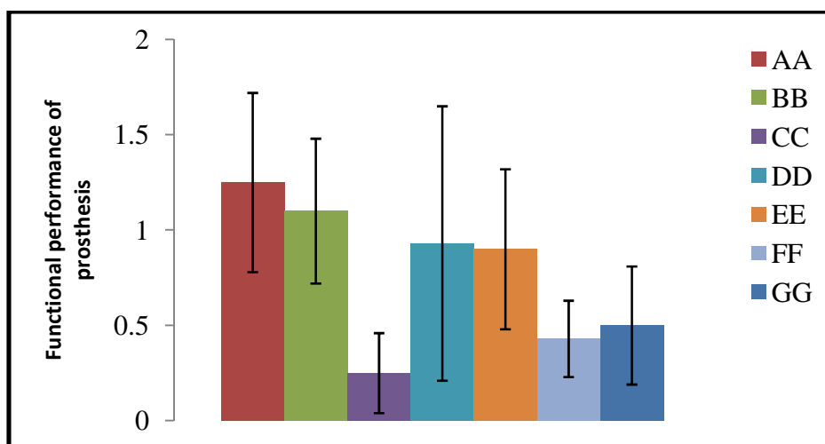
نمودار ۲. میزان موفقیت افراد آمپوتنه روی آرنج در انجام فعالیت‌های مختلف
