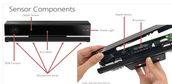
شکل ۱. نمای از حسگر Kinect
